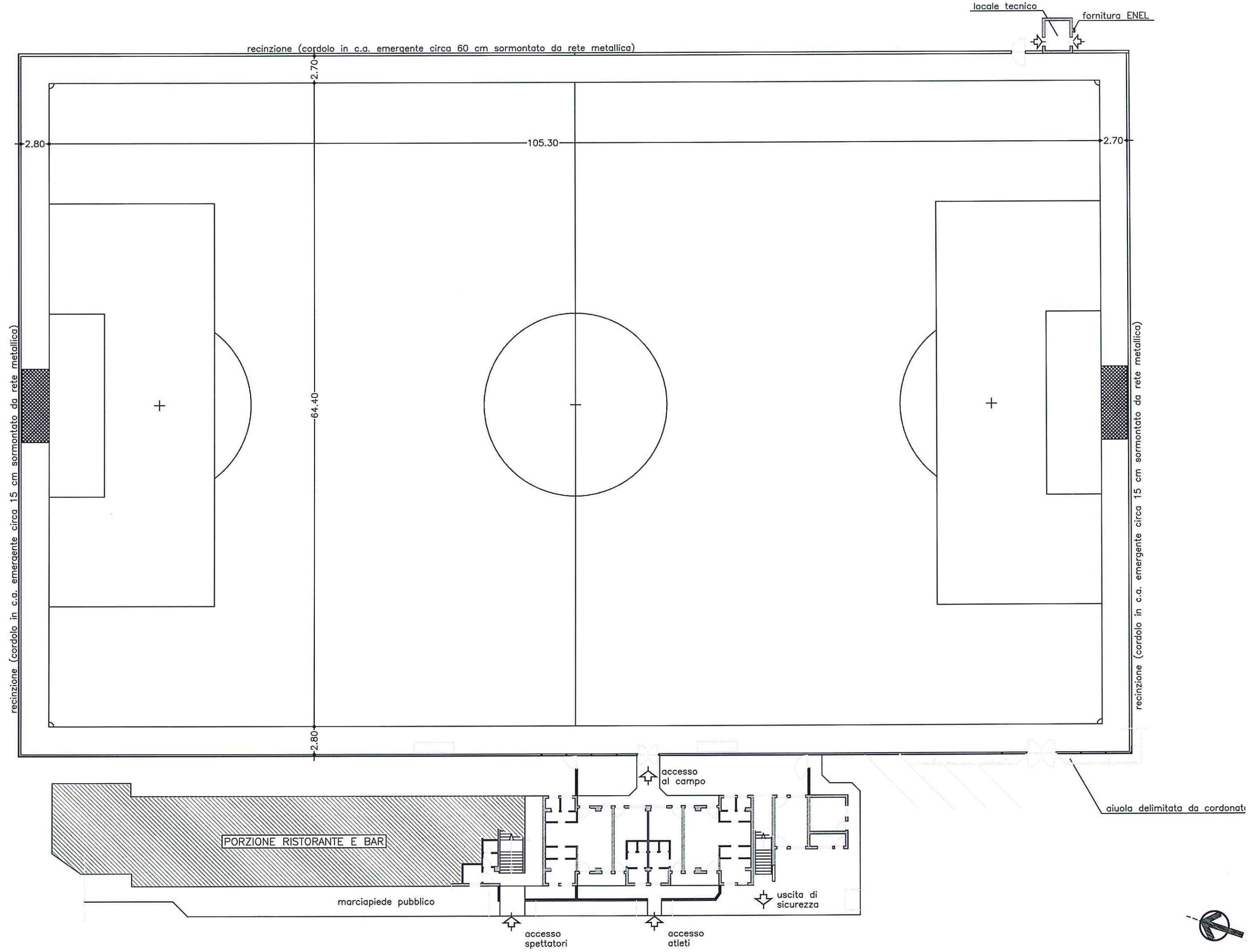
PLANIMETRIA GENERALE DELL'IMPIANTO - SCALA 1:200
